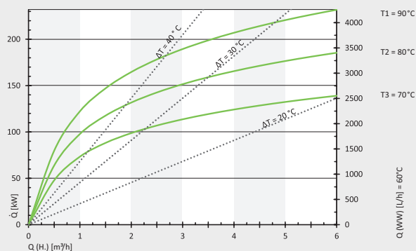
Storatherm Aqua 1500/1 a una temperatura de extracción de 45 °C
