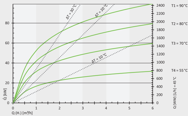
Storatherm Aqua 400/1 a una temperatura de extracción de 60 °C
