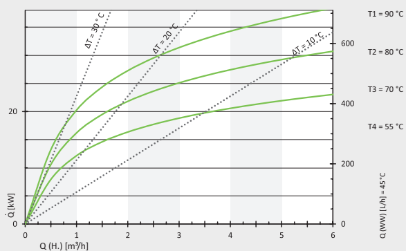
Storatherm Aqua 150/1 a una temperatura de extracción de 60 °C
