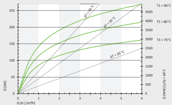
Storatherm Aqua 2000/1 a una temperatura de extracción de 45 °C
