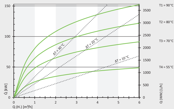
Storatherm Aqua 750/1 a una temperatura de extracción de 45 °C
