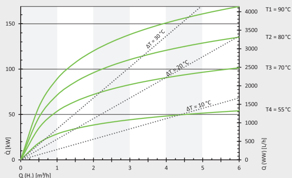
Storatherm Aqua 1000/1 a una temperatura de extracción de 45 °C
