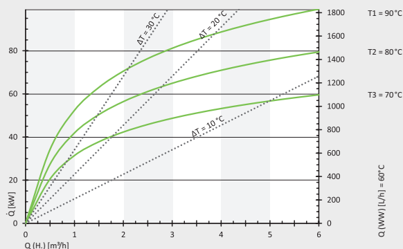
Storatherm Aqua 500/1 a una temperatura de extracción de 60 °C
