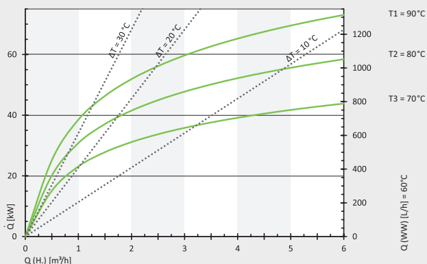
Storatherm Aqua 300/1 a una temperatura de extracción de 60 °C
