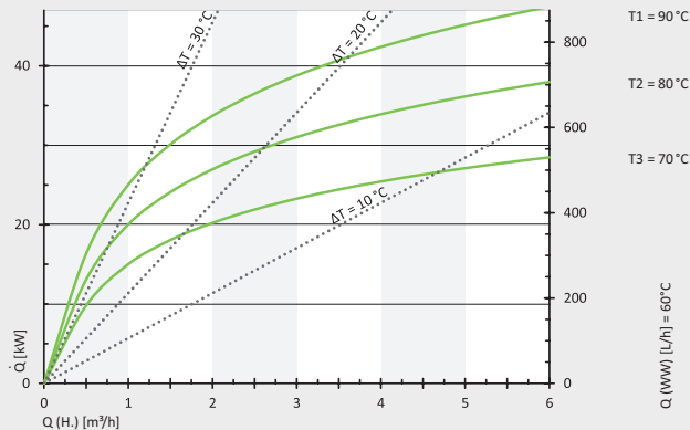
Storatherm Aqua 200/1 a una temperatura de extracción de 60 °C
