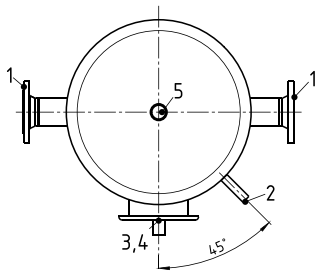
Darstellung ohne Isolation/ Shown without isolation
