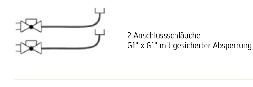
Variomat Anschlüsse für Einpumpenanlage
