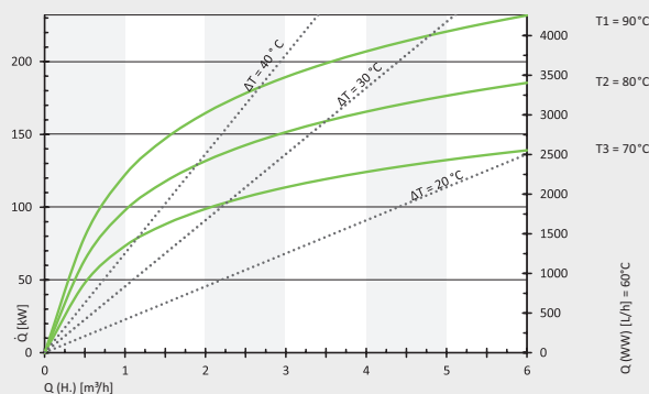
Storatherm Aqua 1500/1 pri teplote odberu 45 °C
