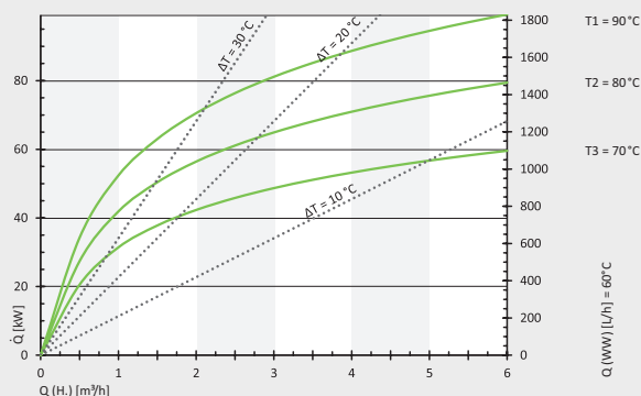
Storatherm Aqua 500/1 pri teplote odberu 60 °C
