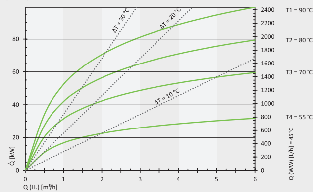
Storatherm Aqua 400/1 pri teplote odberu 60 °C
