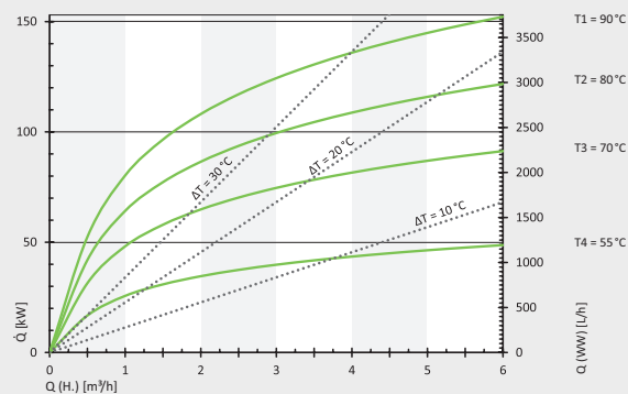
Storatherm Aqua 750/1 pri teplote odberu 45 °C
