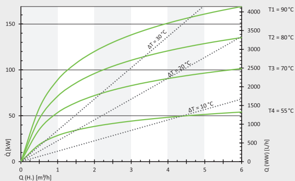
Storatherm Aqua 1000/1 pri teplote odberu 45 °C
