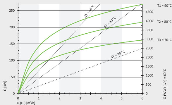
Storatherm Aqua 2000/1 pri teplote odberu 45 °C
