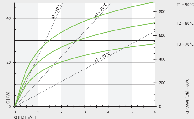
Storatherm Aqua 200/1 pri teplote odberu 60 °C
