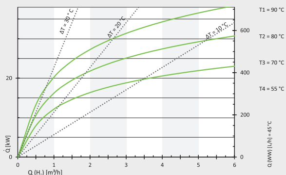
Storatherm Aqua 150/1 pri teplote odberu 60 °C
