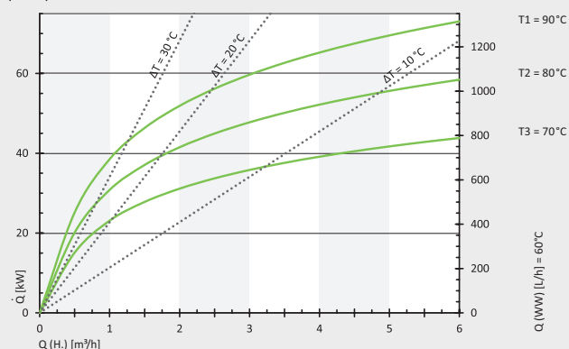
Storatherm Aqua 300/1 pri teplote odberu 60 °C
